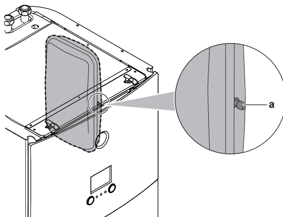
a Schraderjev ventil
