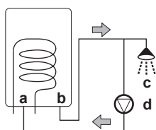
a Priključek za recirkulacijo b Priključek za toplo vodo
