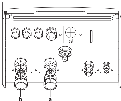
a Штуцер для впуска воды b Штуцер для выпуска воды
