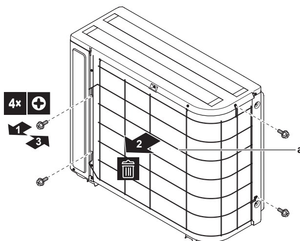
a Решетка воздухозаборника
