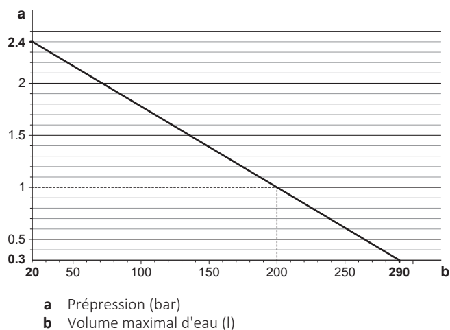
Exemple: volume maximal d'eau et pr  ression du vase d'expansion
