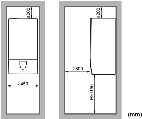
H Hauteur mesurée du bas du boîtier jusqu'au sol
