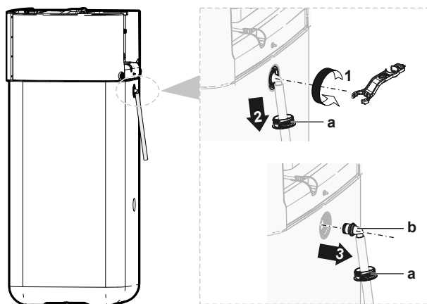
a Spillover-kontakt b Skruvplugg
