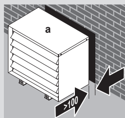
a Poklopac za utišanje zvuka
