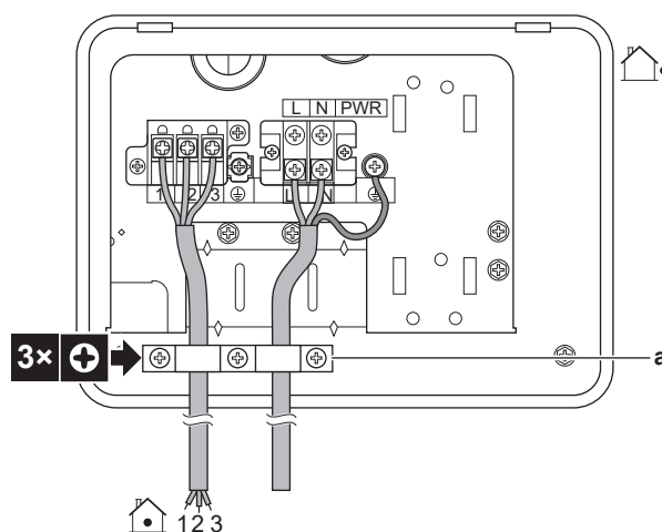
a Кабелна скоба
