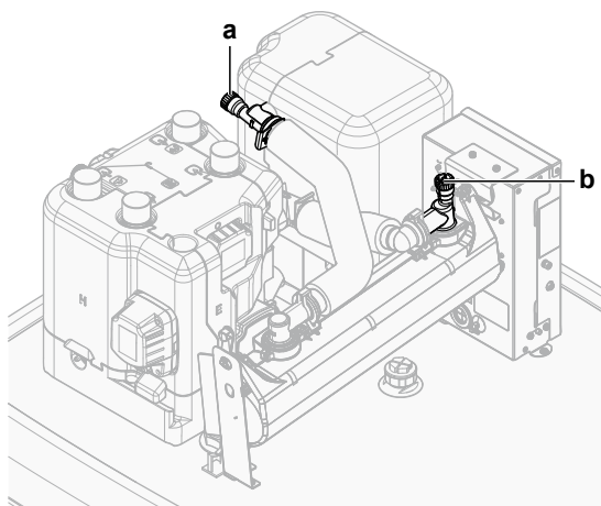
a, b Ръчен вентил на отворите за излизане на въздуха
