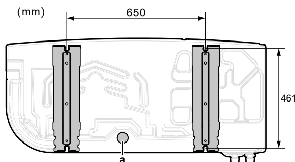
а Дренажное отверстие
