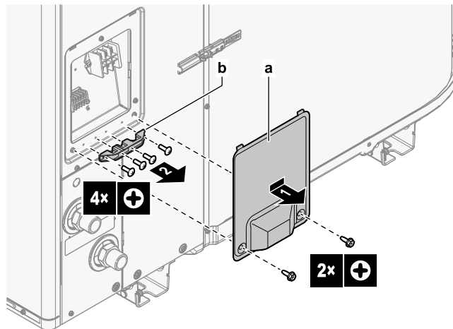
a Pārsegs b Vadu turētājs
