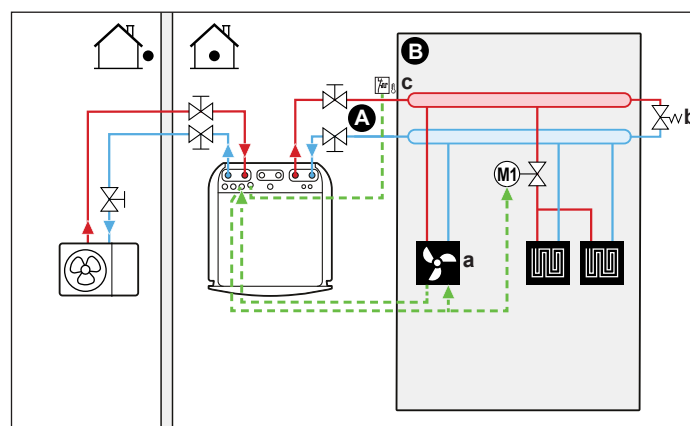
A Haupt-Vorlauftemperaturzone B Ein einzelner Raum
