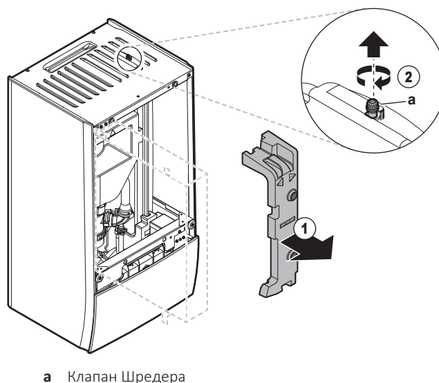
а Клапан Шредера
