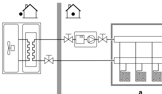
а Основная зона температуры воды на выходе
