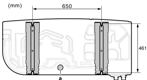
a Дренажное отверстие
