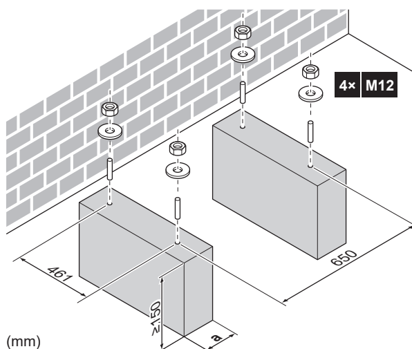
a Обратите внимание, чтобы не был перекрыт доступ к дренажному отверстию в поддоне агрегата.
