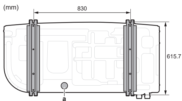
a Дренажен отвор
