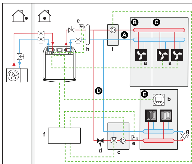
3 Sistema com separador hidráulico para ambas as zonas:
