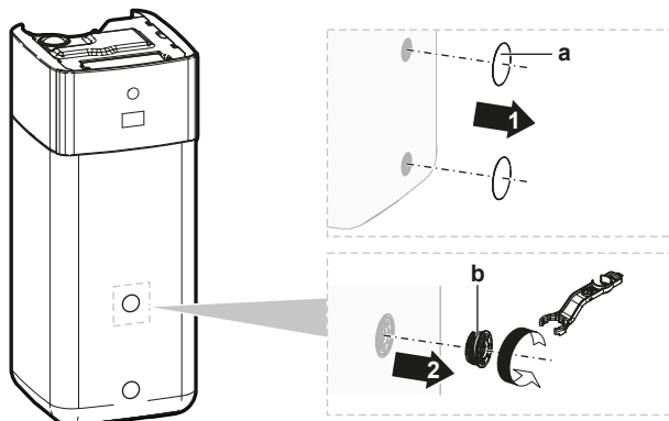
a Couvercle de raccordement b Bouchon à vis
