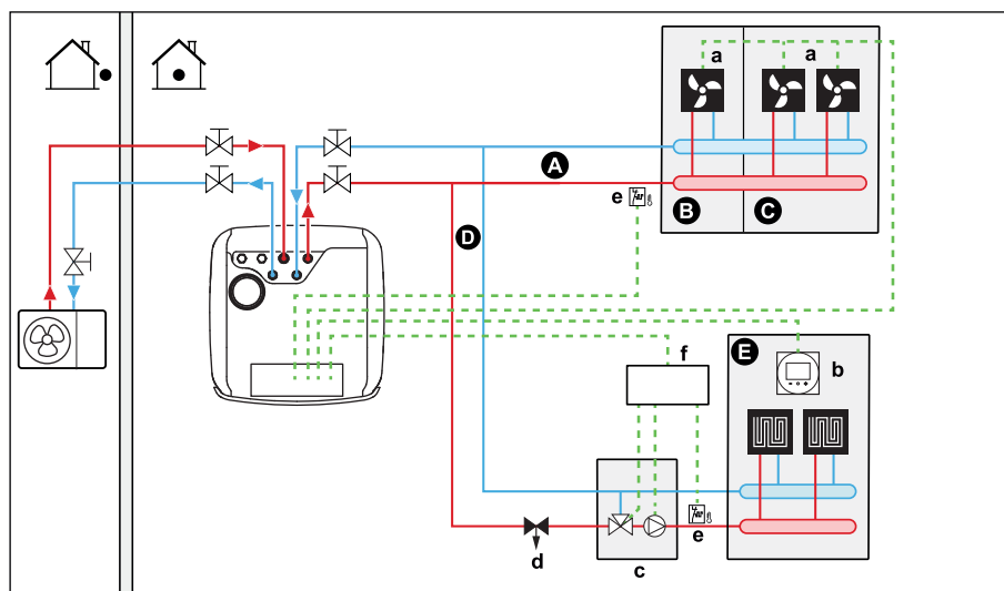
2 System med hydraulisk udskiller til hovedzone:
