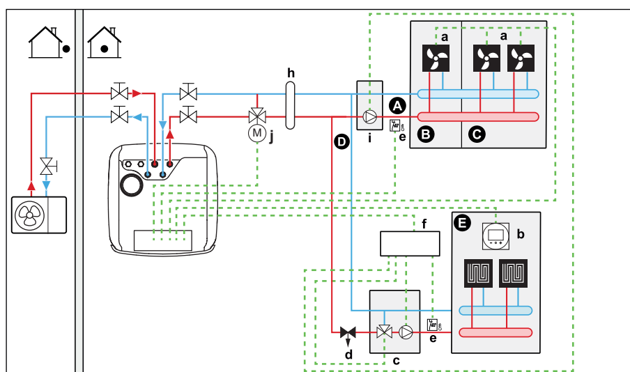
3 System med hydraulisk udskiller til begge zoner:
