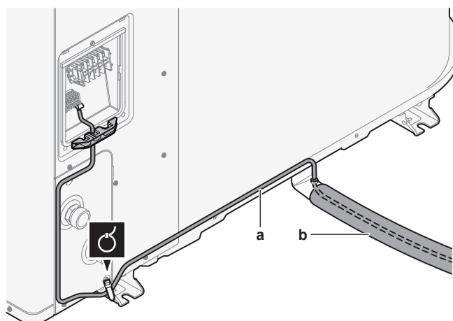
a Kabel til afløbsrørsvarmer b Afløbsrør
