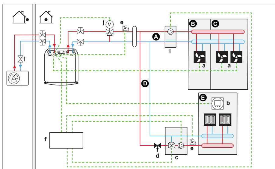
3 Sistem cu separator hidraulic pentru ambele zone: Pentru acest sistem, este necesară o pompă directă pentru zona suplimentară.
