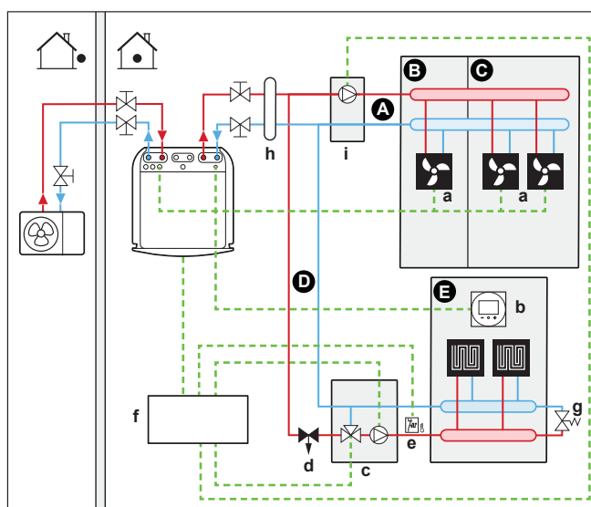
3 Система с хидравличен сепаратор за двете зони: За тази система е необходима директна помпа за допълнителната зона.
