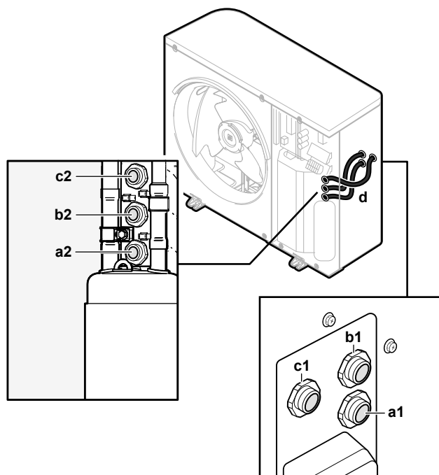
a1+a2 Кабел за захранване с електричество (доставка на място)
