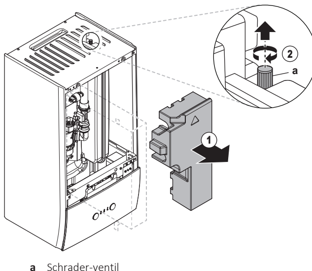
a Schrader-ventil
