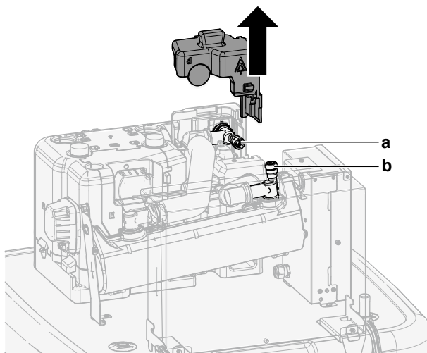
a, b Βάνα χειροκίνητου εξαερισμού
