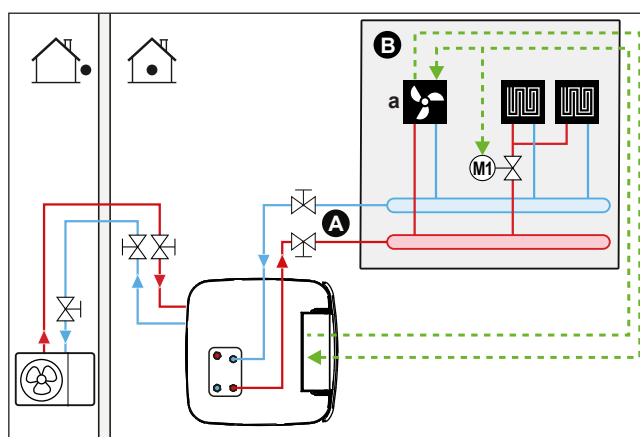
A Κύρια ζώνη θερμοκρασίας εξερχόμενου νερού B Ένας μόνο χώρος
