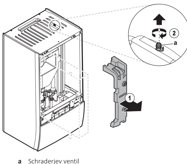
a Schraderjev ventil
