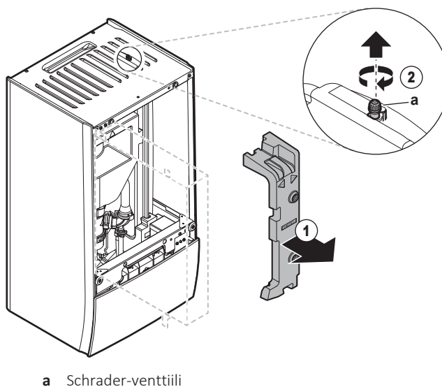
a Schrader-venttiili
