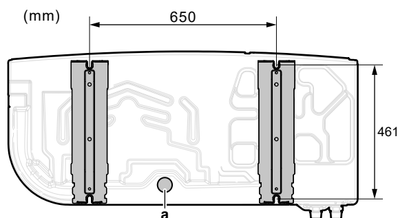
a Tyhjennysaukko
