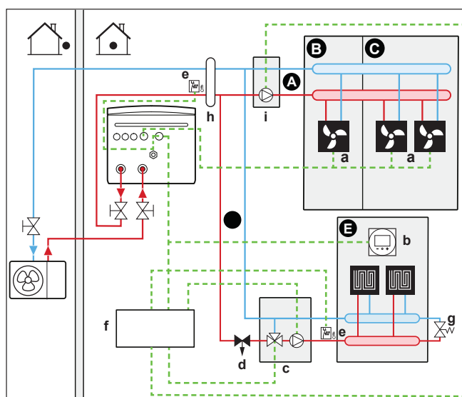
3 Sistema amb separador hidràulic per a ambdues zones:
