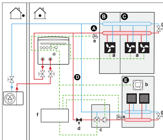
2 Sistema amb separador hidràulic per a la zona principal:
