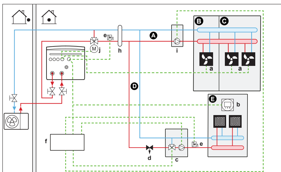
3 Système avec séparateur hydraulique pour les deux zones:
