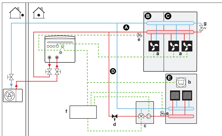
2 Σύστημα με υδραυλικό διαχωριστή για την κύρια ζώνη:
