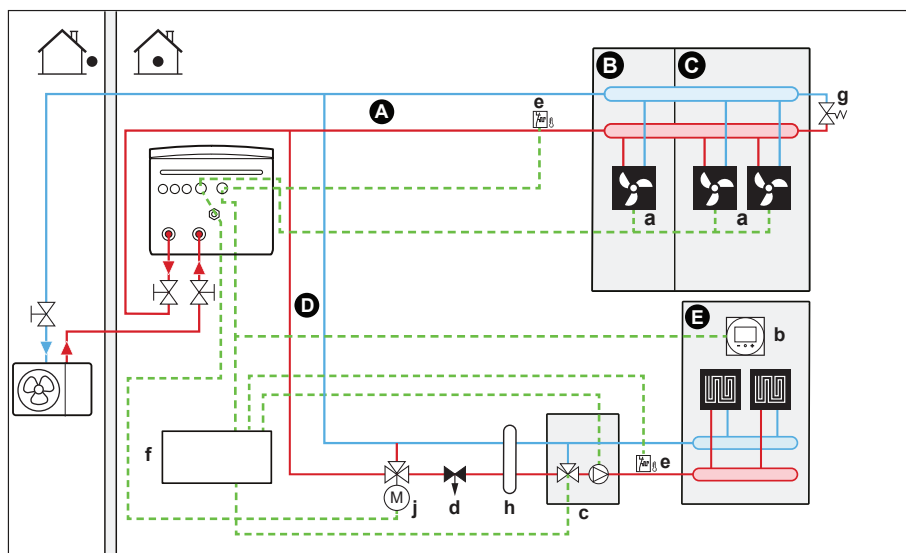
3 Σύστημα με υδραυλικό διαχωριστή και για τις δύο ζώνες:
