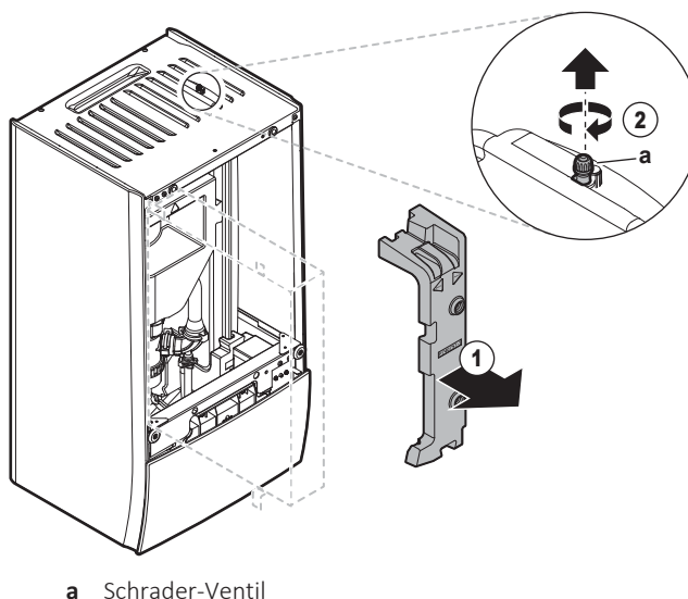
a Schrader-Ventil
