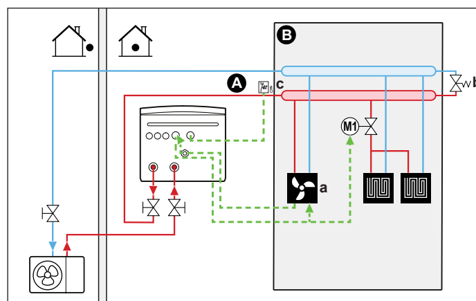
A Haupt-Vorlauftemperaturzone
