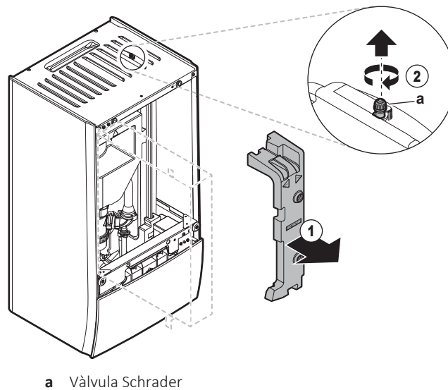
a Vàlvula Schrader
