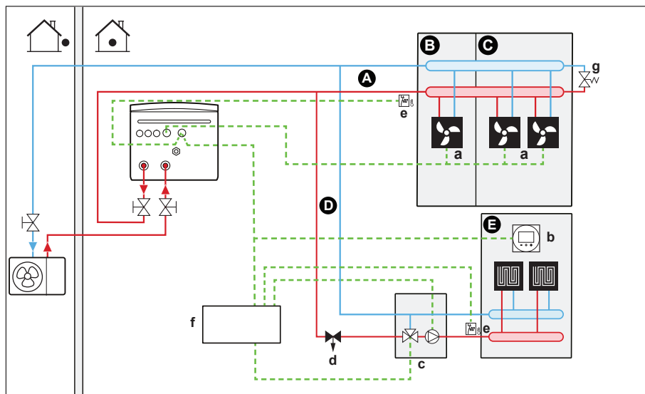
2 Система с хидравличен сепаратор за основната зона:
