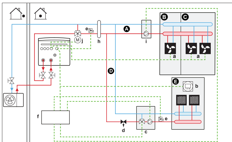
3 Система с хидравличен сепаратор за двете зони:
