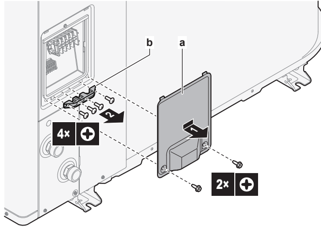
a Kapak b Kablo tutucu
