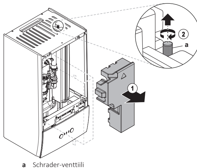
a Schrader-venttiili
