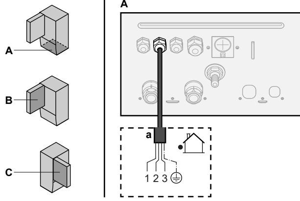
a Ara bağlantı kablosu (=ana güç kaynağı)
