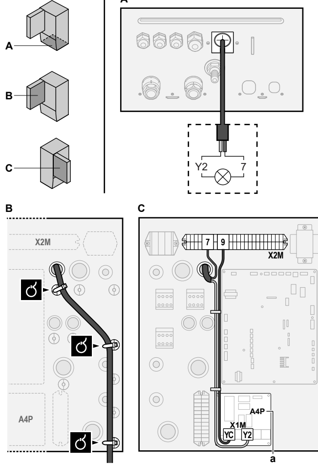
a EKRP1HBAA monte edilmesi gerekir.
