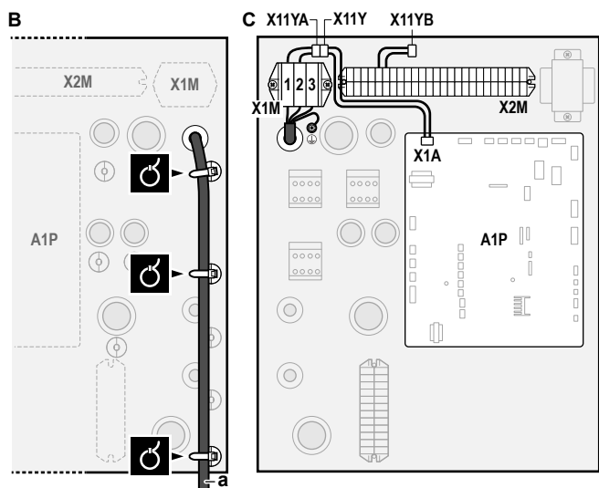
a Соединительный кабель (=основное электропитание)
