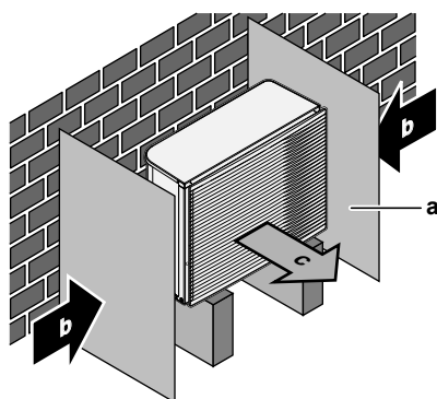
a Защитная панель b Преобладающее направление ветра c Выброс воздуха
