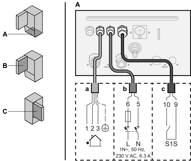
a Соединительный кабель (=основное электропитание) b Источник электропитания по обычному тарифу c Контакт подачи электропитания с предпочтительным энергосбережением
