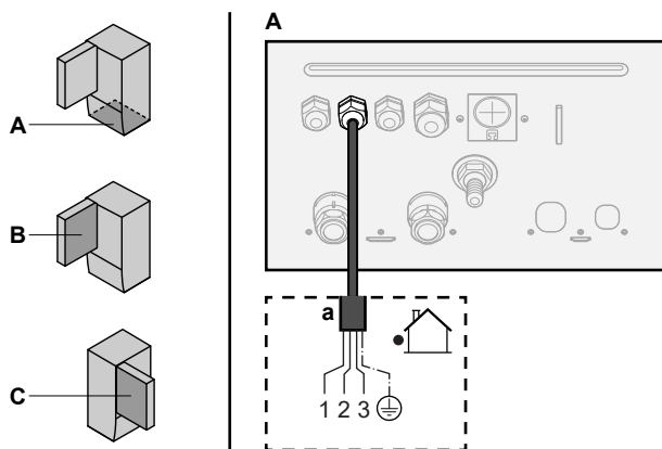
a Соединительный кабель (=основное электропитание)
