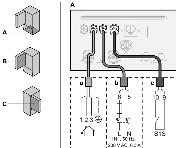
a Kabel połączeniowy (=główne zasilanie) b Zasilanie z taryfą o normalnej stawce kWh c Styk zasilania o korzystnej stawce
