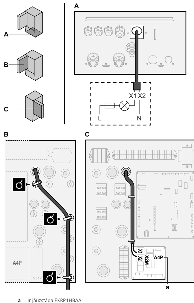
a Ir jāuzstāda EKR1HBAA.
