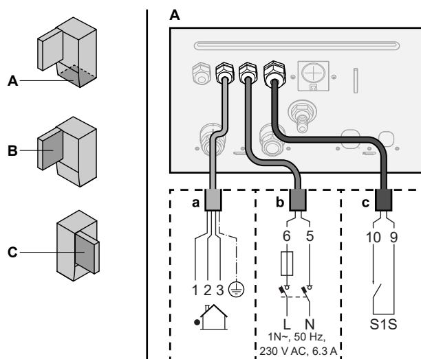
a Starpsavienojuma kabelis (=strāvas padeve) b Normāla kWh nomināla strāvas padeve c Vēlamais strāvas padeves kontakts
