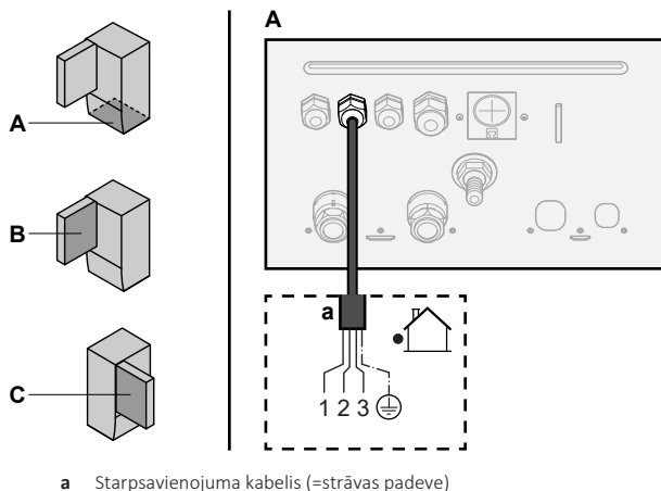
a Starpsavienojuma kabelis (=strāvas padeve)
