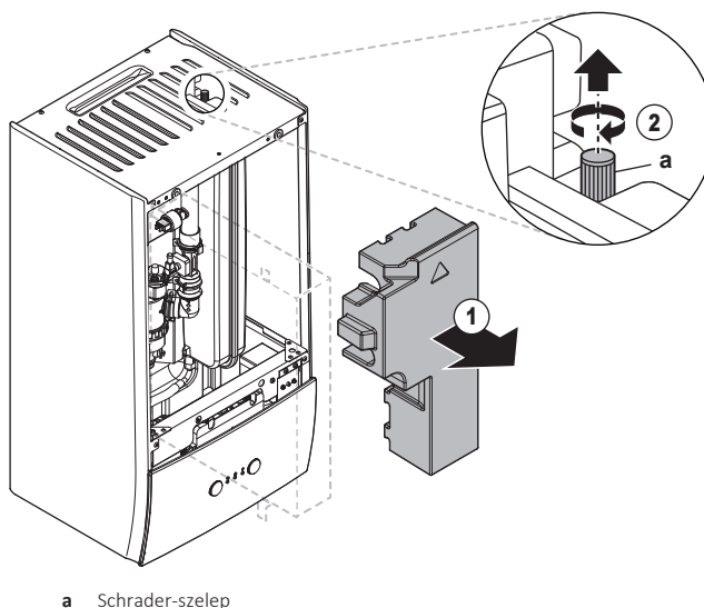
a Schrader-szelep
