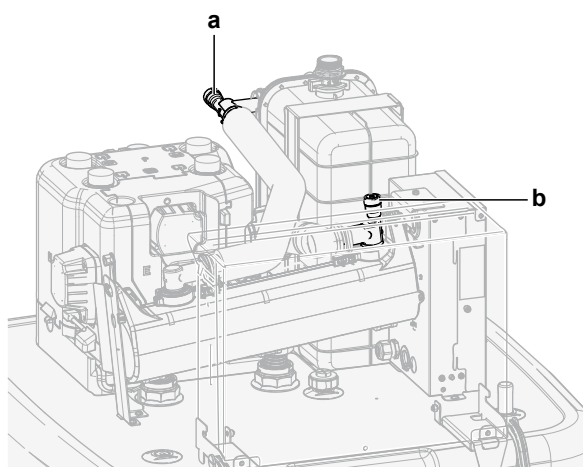
a, b Manuell luftningsventil
