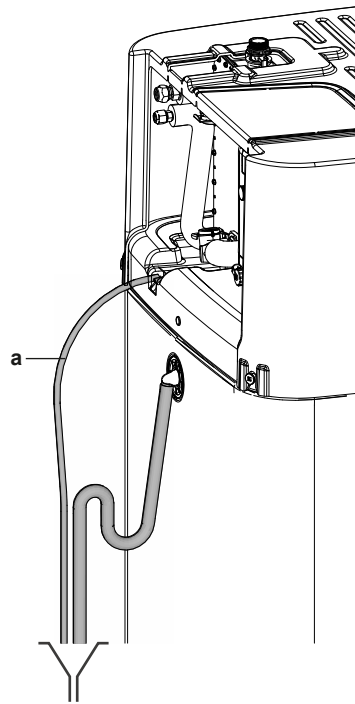
a Dräneringstrågets slang
