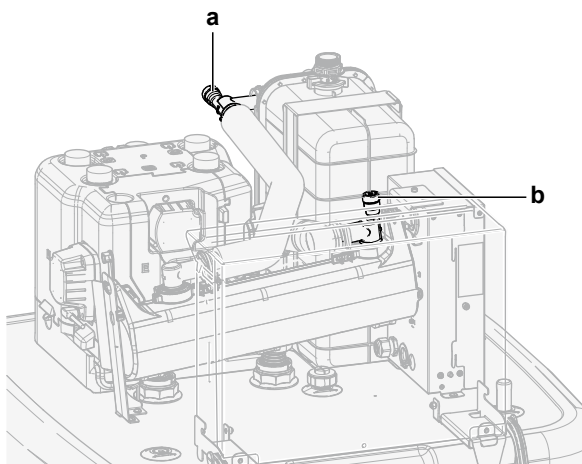
a, b Manuálny odvzdušňovací ventil
