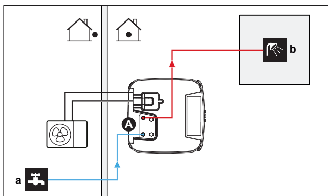
A Nádrž teplej vody pre domácnosť
