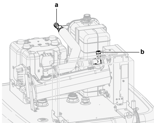
a, b Ruční odvzdušňovací ventil
