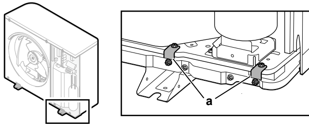
a Prepravné podpery (2x)
