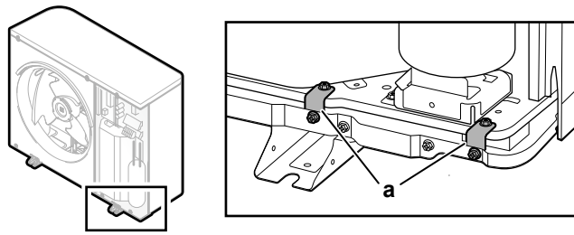
a Soportes de transporte (2x)
