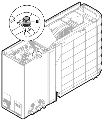
a Schraderjev ventil
