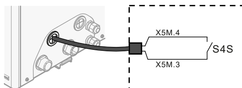
S4S Impulzni števec za pametno električno omrežje (opcijski)
