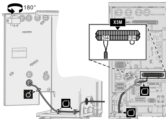
S4S Impulzni števec za pametno električno omrežje (opcijski)
