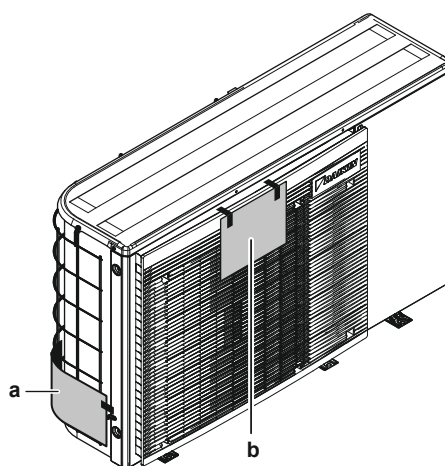
a Ochranný kartón b Hárrok s pokynmi
