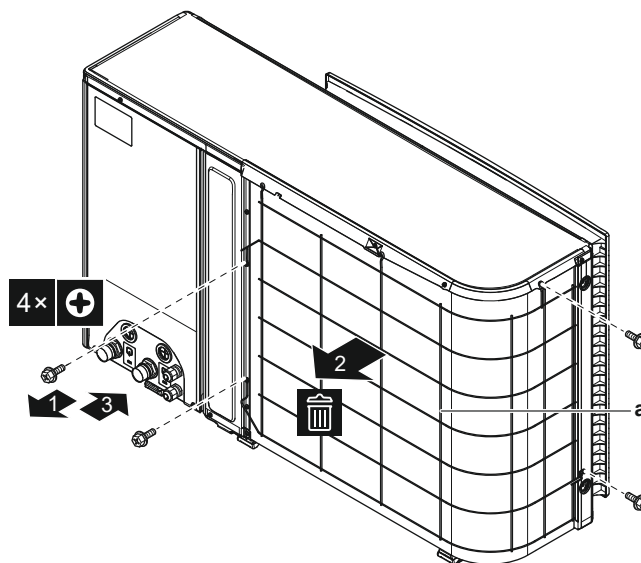
a Mriežka nasávania
