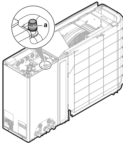
a Βαλβίδα Schrader
