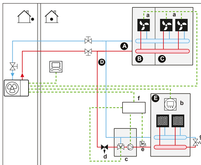
2 Система с хидравличен сепаратор за основната зона:
