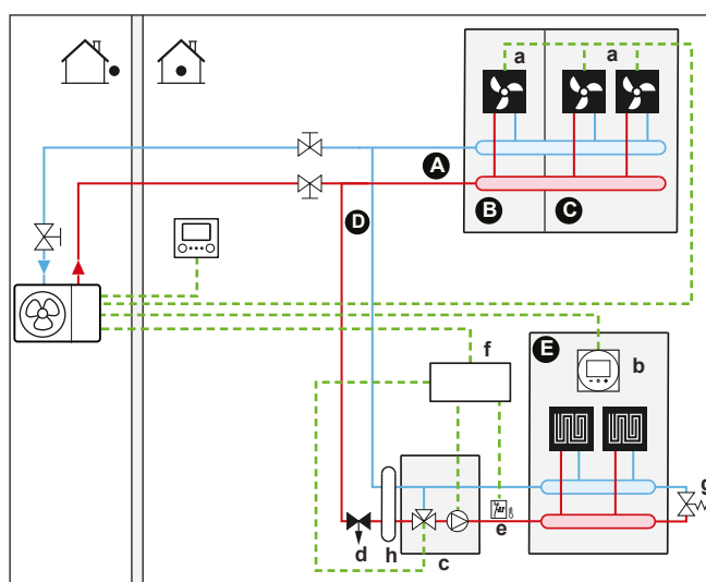
3 Система с хидравличен сепаратор за двете зони:
