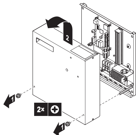
7.2.4 So öffnen Sie den Steuerungskasten
