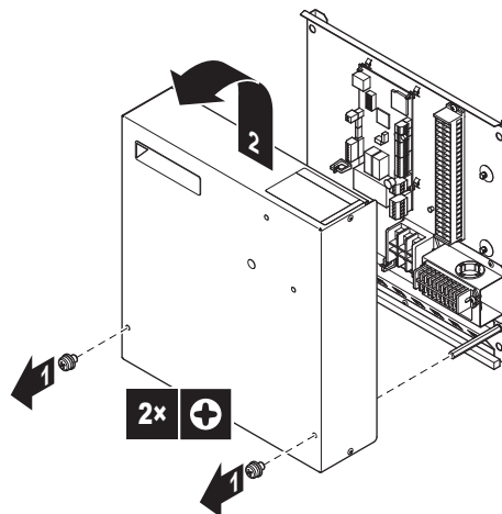
7.2.3 So öffnen Sie die Schaltkastenabdeckung des Außengeräts
