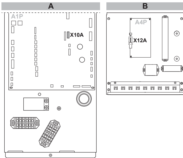
A Schaltkasten des Außengeräts B Schaltkasten des Steuerungskastens
