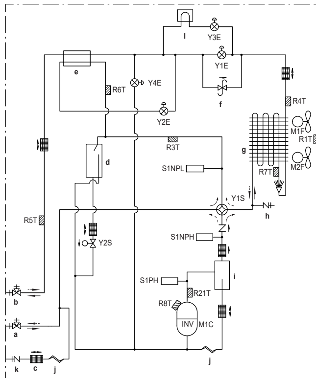
Diagram cevovoda: 10+12 HP
