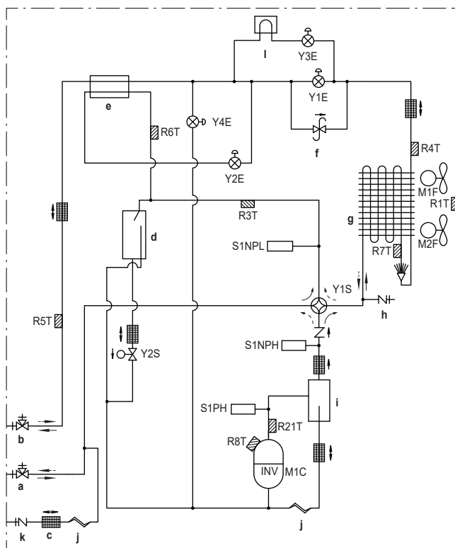
Diagram cevovoda: 10+12 HP
