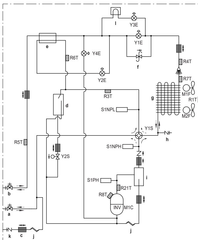
Diagram cevovoda: 10+12 HP
