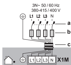
a Zemljistični odklopnik b Varovalka c Kabel za električno napajanje
