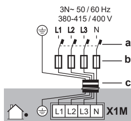
a Автоматический выключатель защиты от замыкания на землю b Плавкий предохранитель c Кабель электропитания
