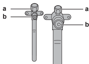
a Сервисное отверстие b Запорный вентиль
