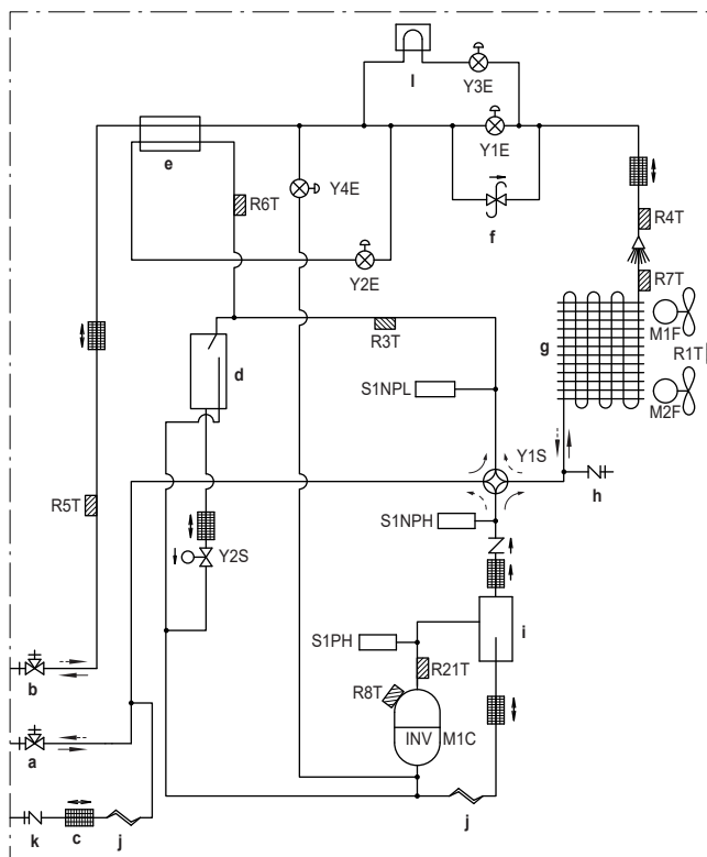
Schema delle tubazioni: 10+12 HP
