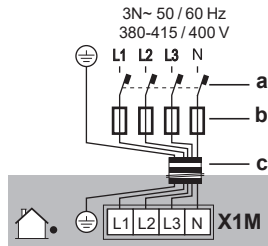
a Maavuotosuojakatkaisin b Sulake c Virransyöttökaapeli
