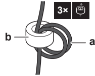
a Yhteiskytkentäkaapeli b Ferriittisydän
