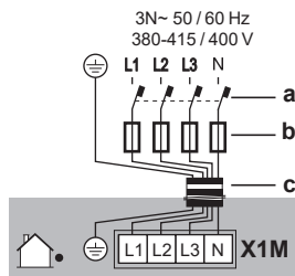
a Ασφαλειοδιακόπτης διαρροής γείωσης b Ασφάλεια c Καλώδιο παροχής ρεύματος
