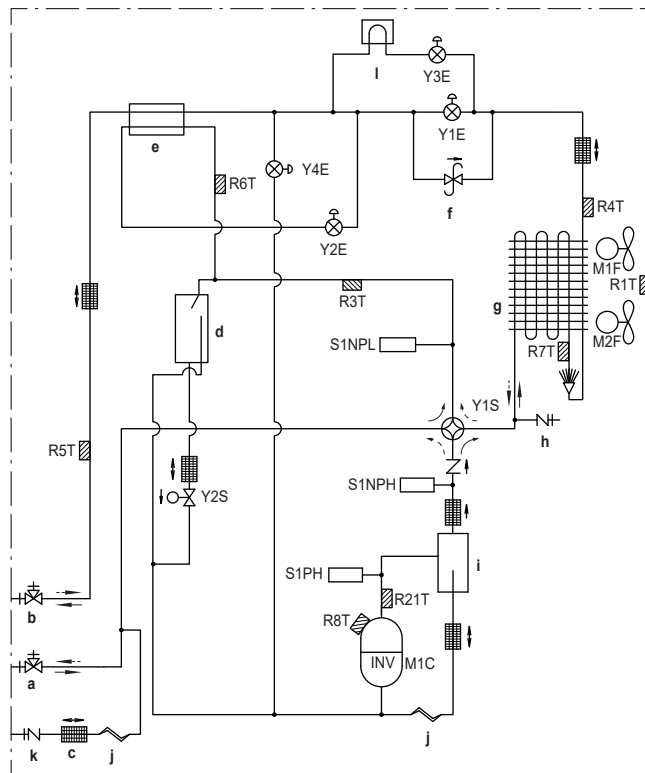
Rohrleitungsplan: 10+12 HP
