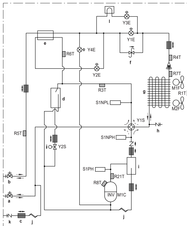
Rohrleitungsplan: 10+12 HP
